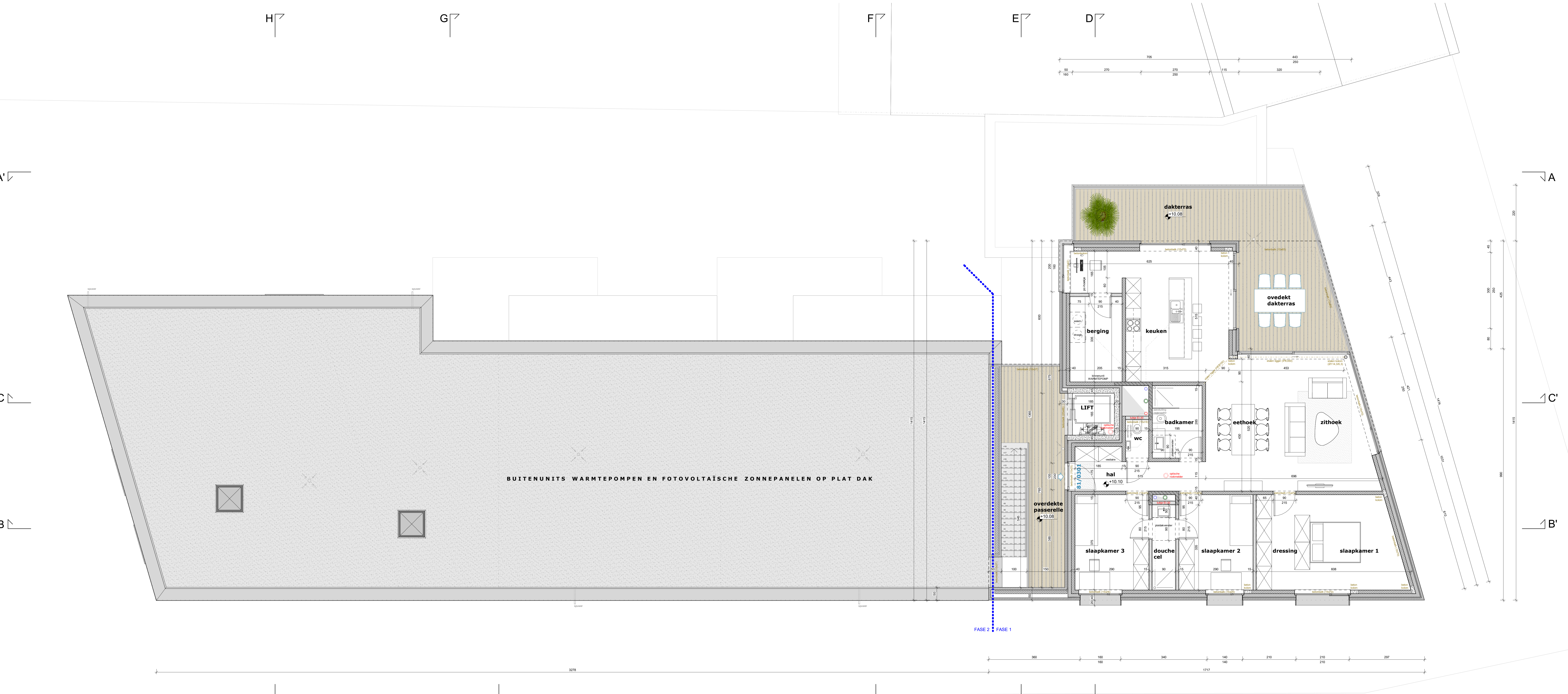
3 Plan verdieping 3 1 : 50
